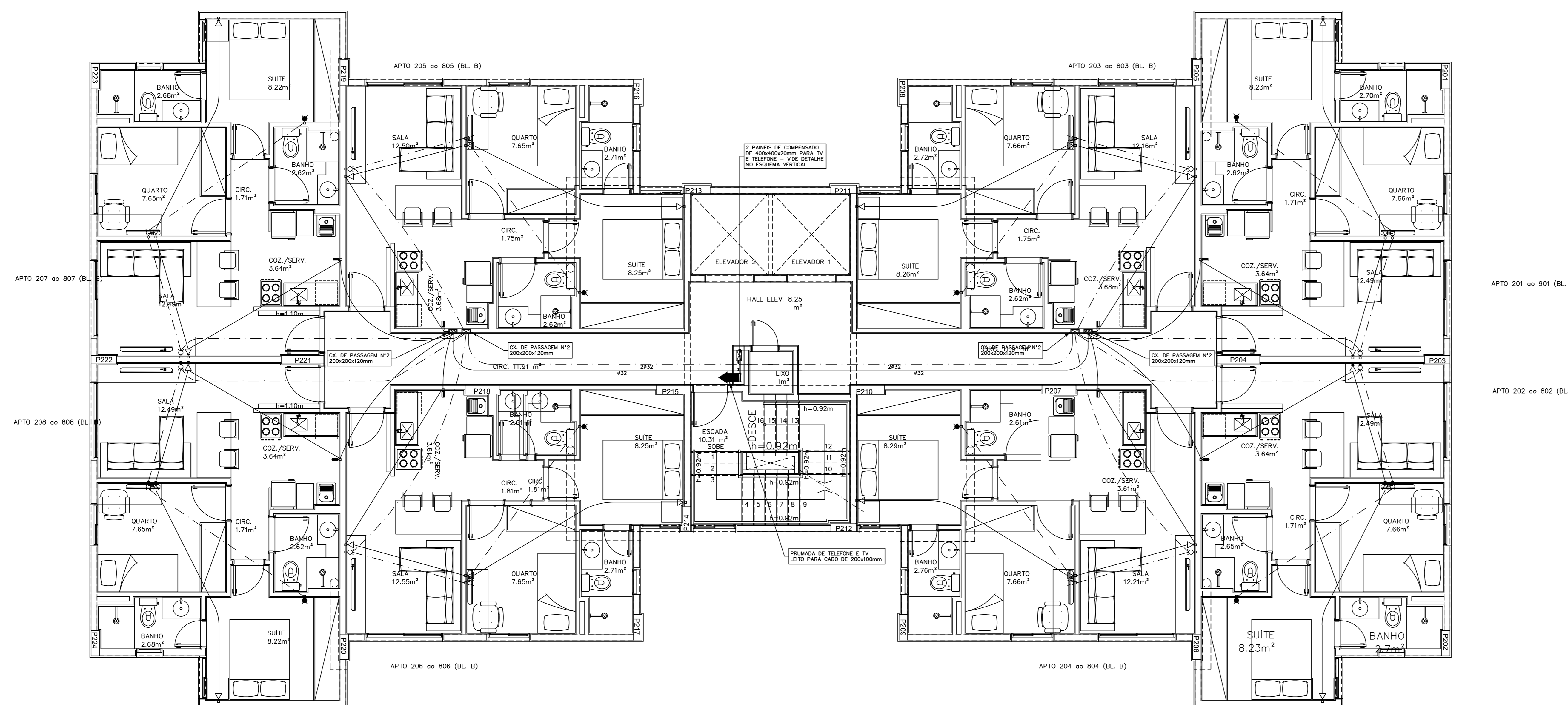
PLANTA BAIXA PAVIMENTO TIPO BLOCO B ESCALA 1:50
