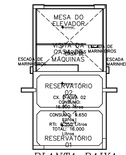
PLANTA BAIXA RESERVATORIO ESCALA 1:100
