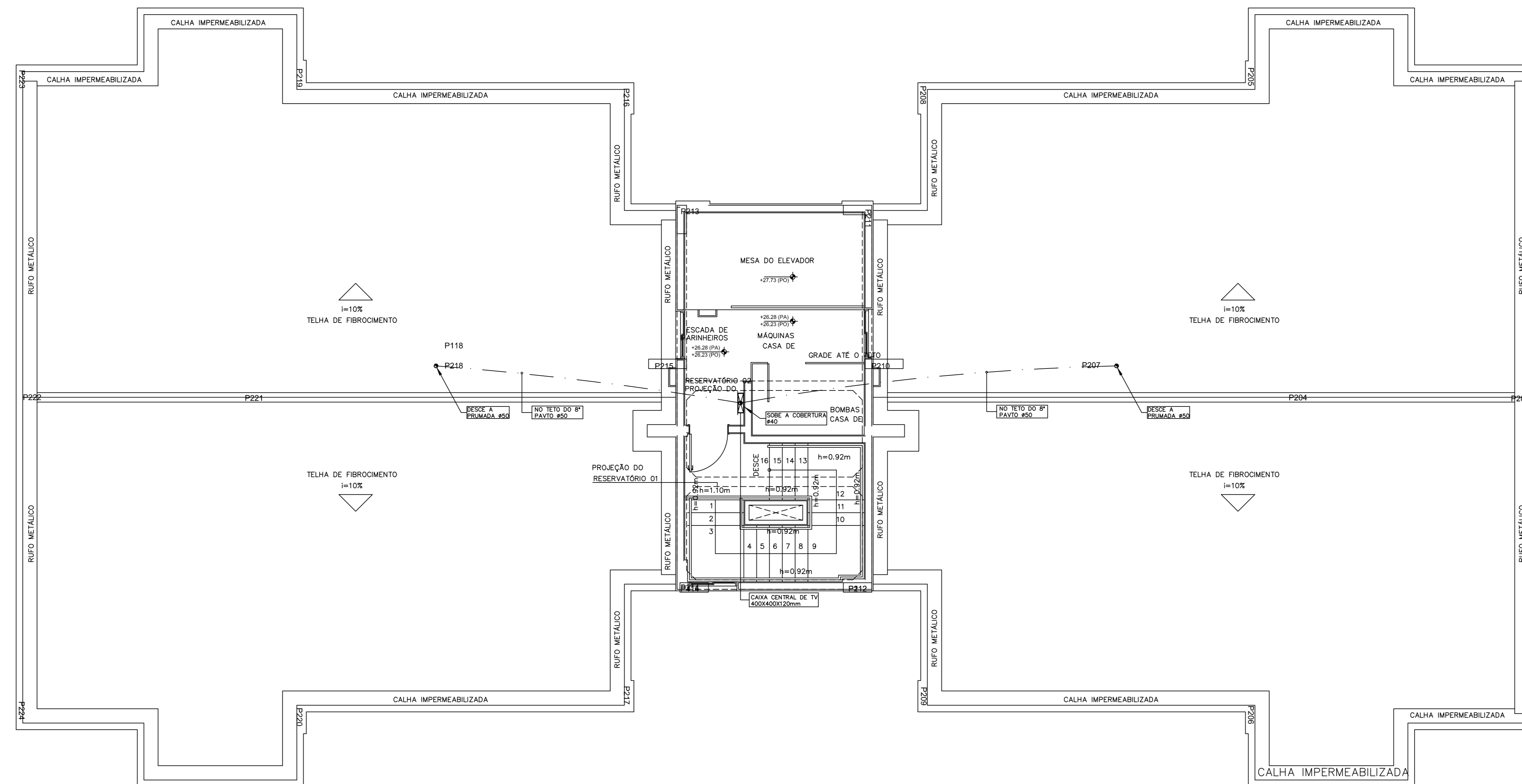
PLANTA BAIXA PAVIMENTO COBERTURA B ESCALA 1:50
