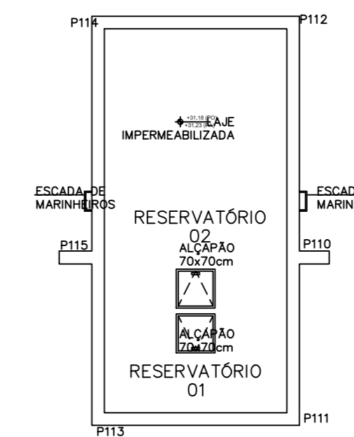
PLANTA BAIXA CX. D'ÁGUA ESCALA 1:100
